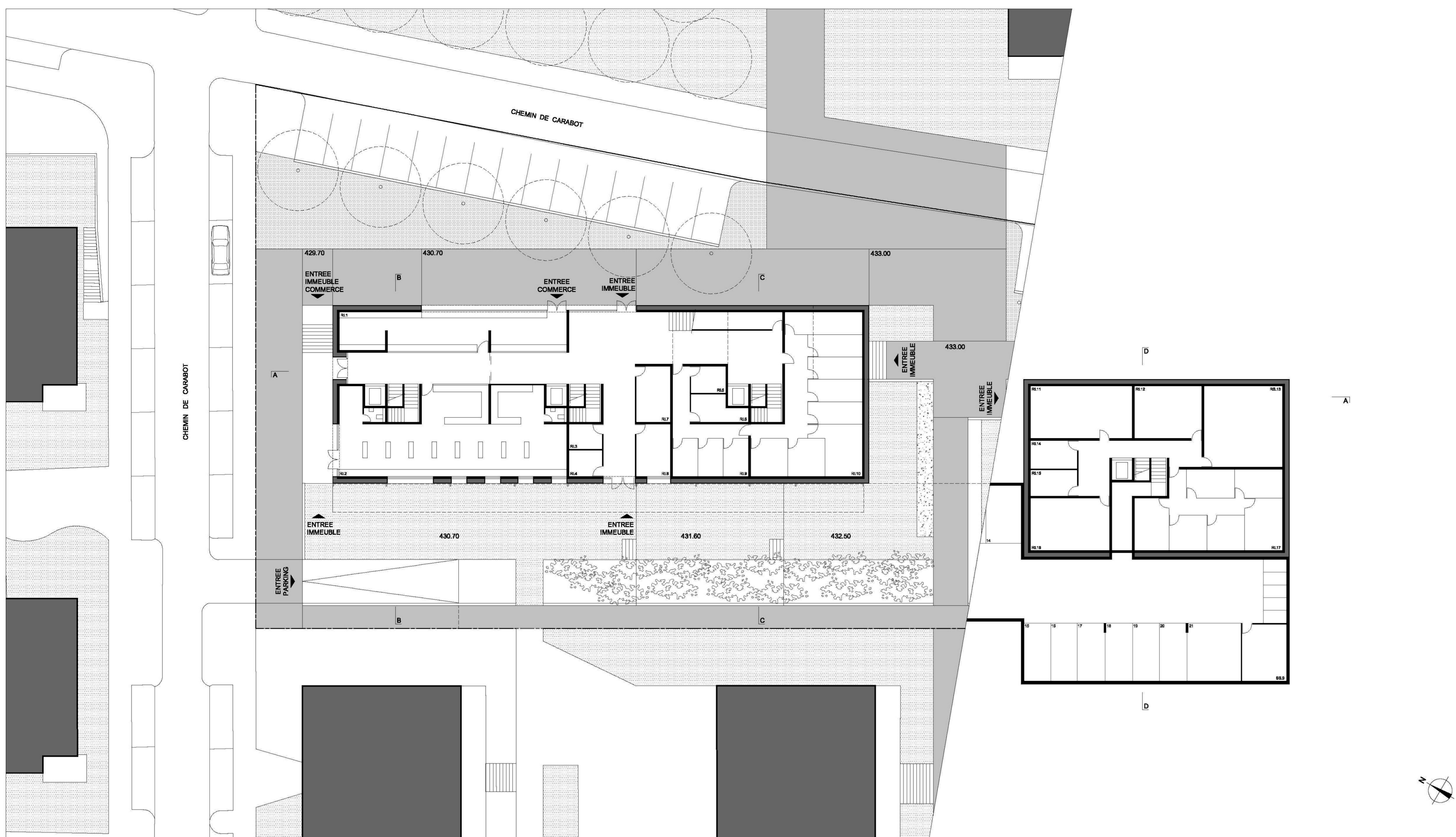
REZ-DE-CHAUSSEE INFERIEUR (ECH. 1/200)
