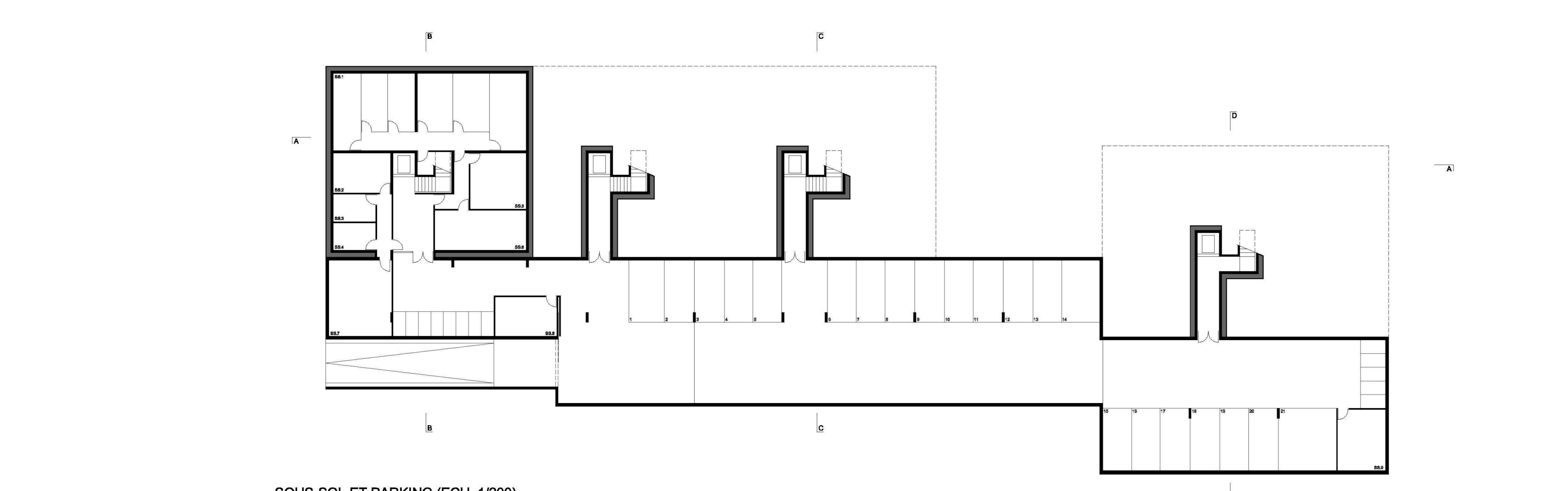
SOUS-SOL ET PARKING (ECH. 1/200)
