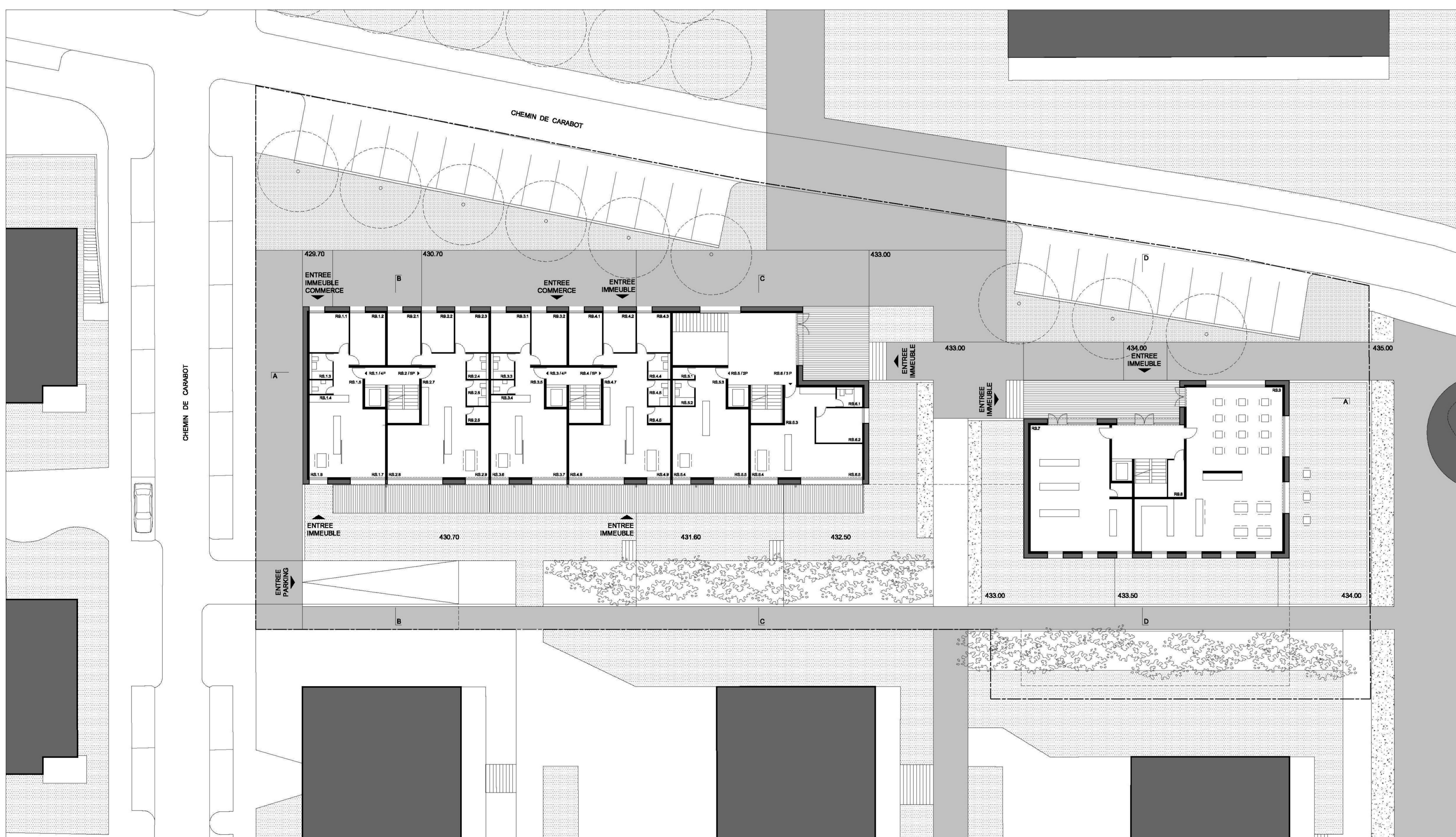
REZ-DE-CHAUSSEE SUPERIEUR (ECH. 1/200)
